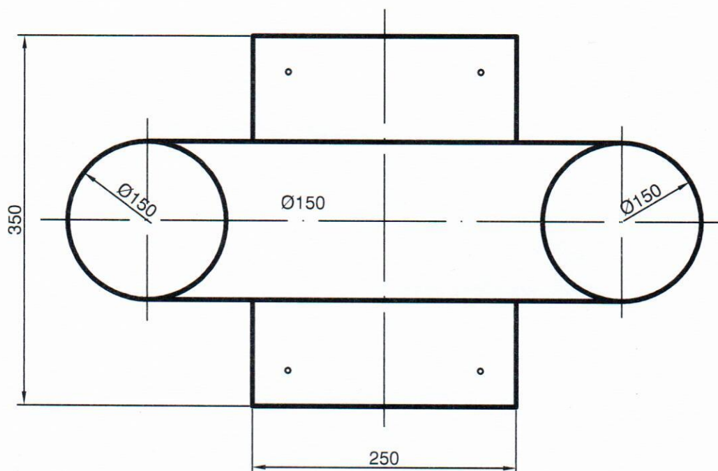
Nasada typu H \text{Ø}150\text{mm} z ramionami cylindrycznymi i płytą kominową
